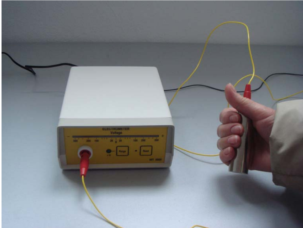
Foto 10 Aparat pentru măsurarea încărcării electrostatice a persoanelor
