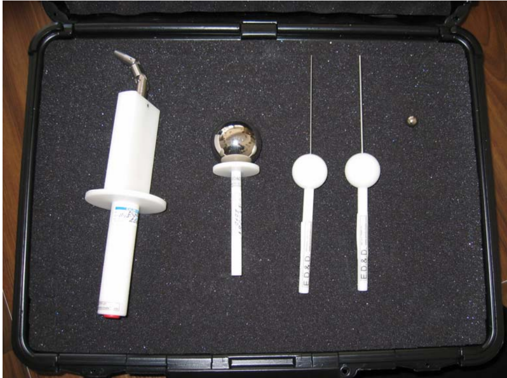
Figura 5. Trusa de calibre de acces
